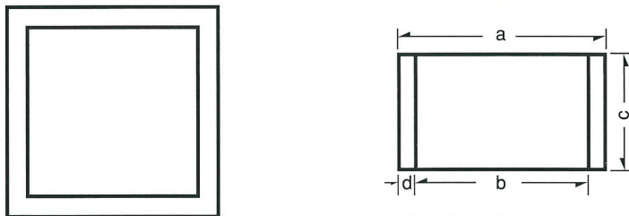
ツギ桧寸法および重量表
