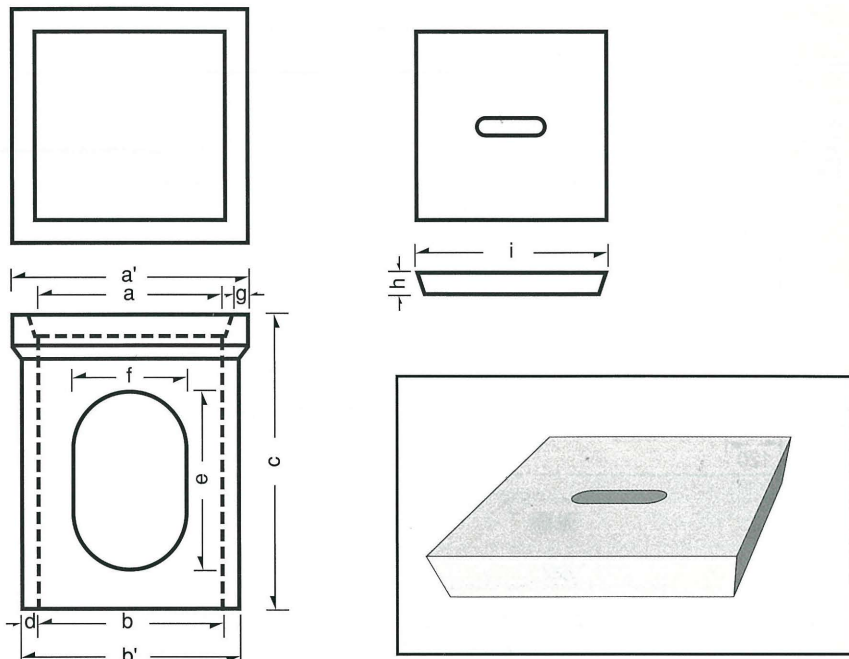
溜桧寸法および重量表
