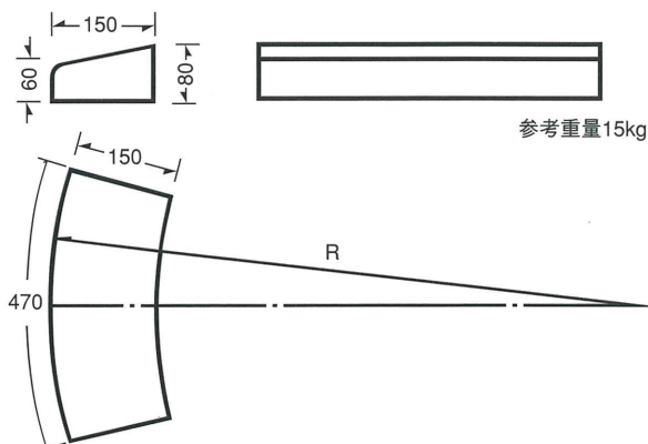
L型街渠用ブロックB型（曲）切下平
