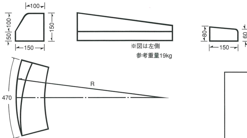
L型街渠用ブロックB型（曲）切下斜
