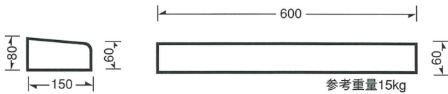
L型街渠用ブロックB型（直）切下平
