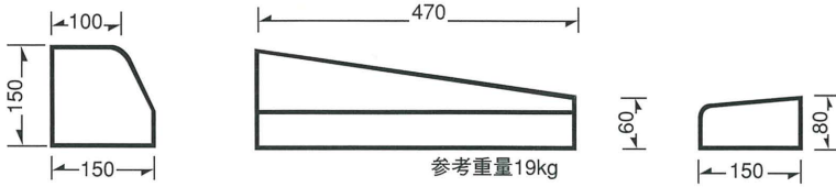
L型街渠用ブロックB型（直）切下斜 L=470
