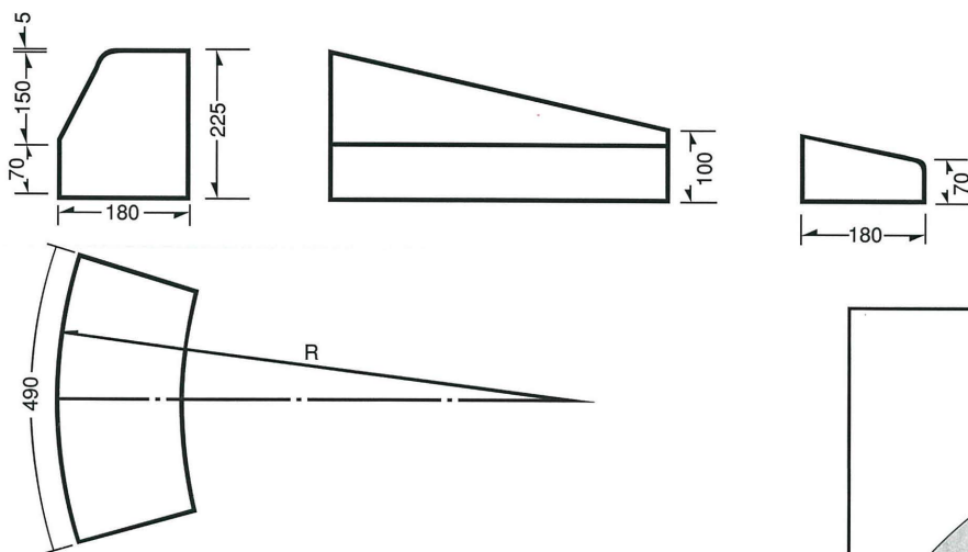
L型街渠用ブロックA (曲) 切下斜
