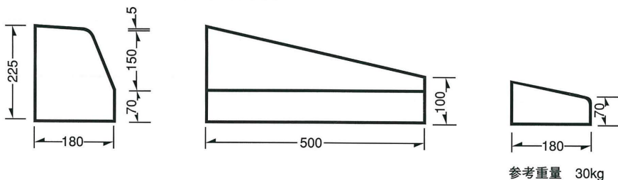
L型街渠用ブロックA (直) 切下平
