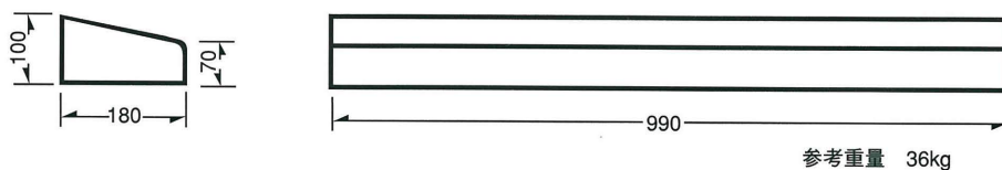
L型街渠用ブロックA (曲) 切下斜
