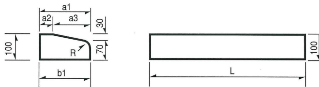
身障者用歩車道境界ブロック切下げ平
