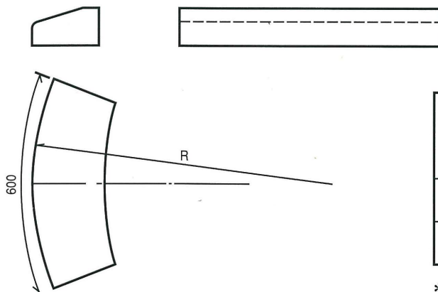
身障者用歩車道境界ブロック切下げ平曲り
