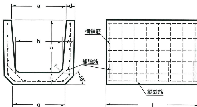
鉄筋コンクリートU形 (呼び名240以上)
