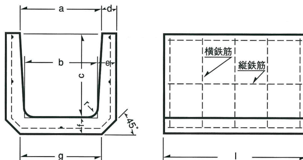
鉄筋コンクリートU形 (呼び名240以上)
