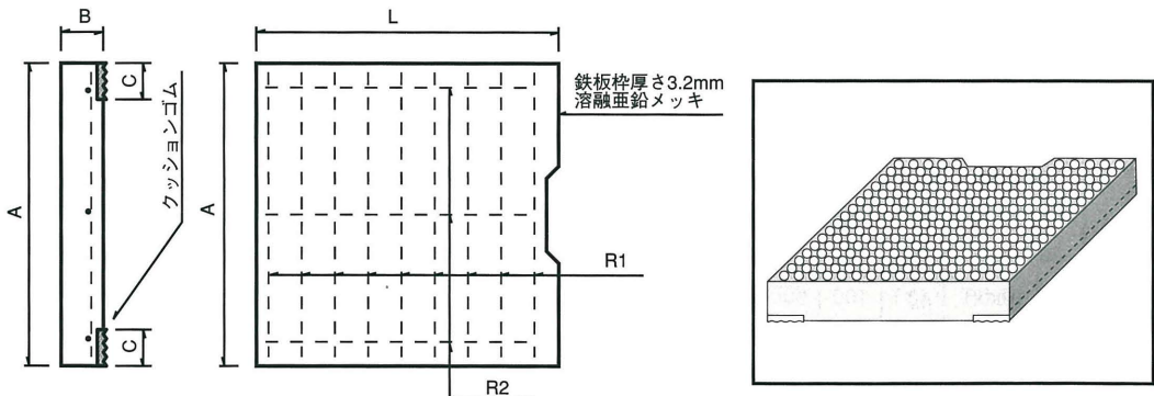
寸法、鉄筋及び重量表
