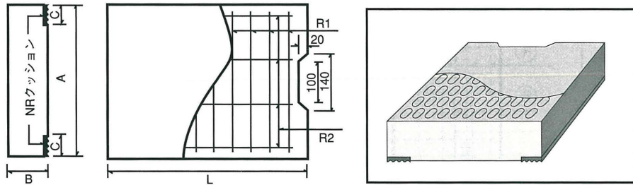
寸法、鉄筋及び重量表
